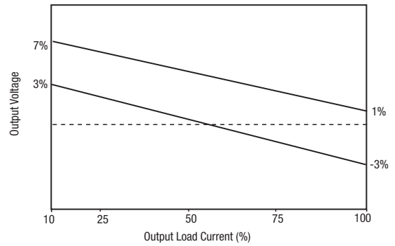
CRE1S0505S3C
