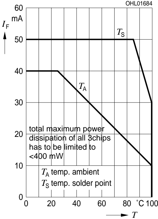
Maximal zulässiger Durchlassstrom blau Max. Permissible Forward Current blue I_F = f(T) ; 3 chips on
