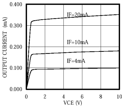
I_o vs V_{CE}
