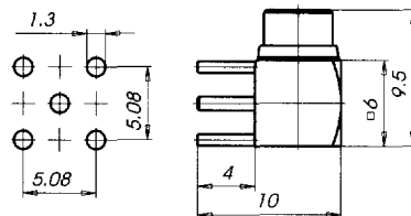
Montagebohrungen Mounting Detail
