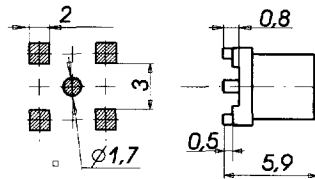
SMT-Lötflächen Solderpad Layout
