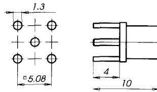
Montagebohrungen Mounting Detail
