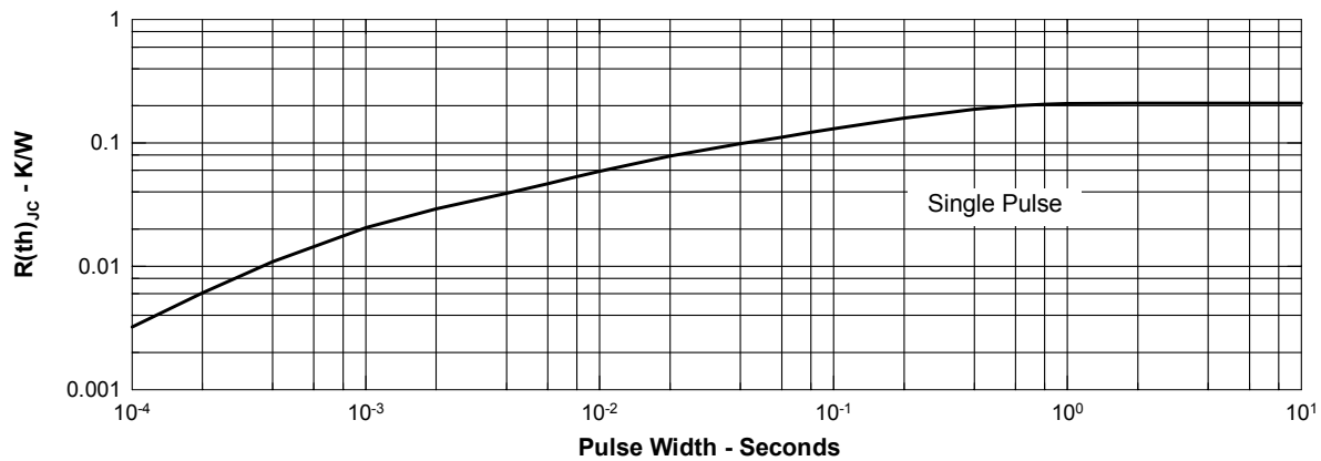
Fig. 10. Thermal Impedence
