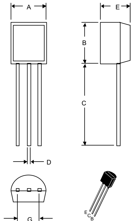
DIMENSIONS
