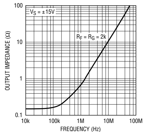
LT1259/60 • TPC10
