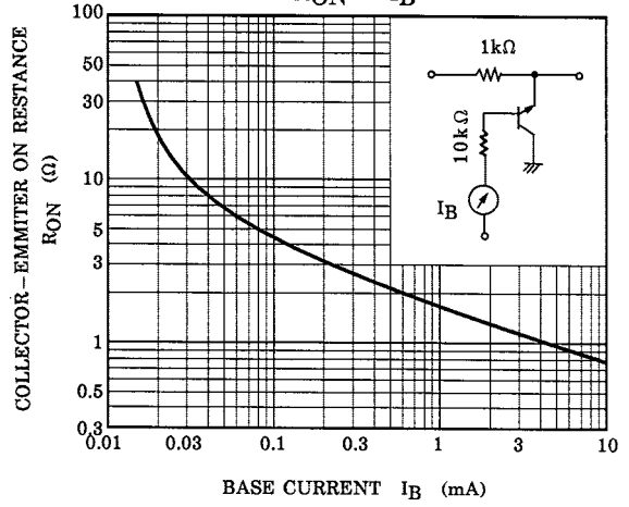
R_{ON} - I_B
