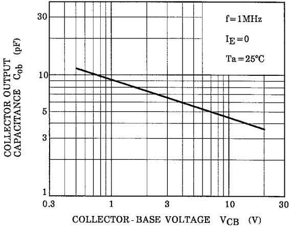
C_{ob} - V_{CB}
