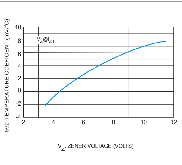
Fig. 2 Zener Voltage - to 12 volts
