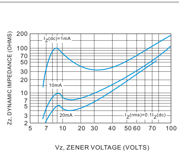
Fig. 5 Effect of Zener Voltage
