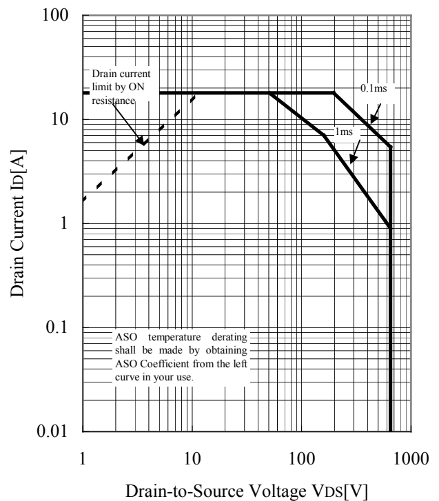
IRIS-X6757 MOSFET A.S.O. Curve
