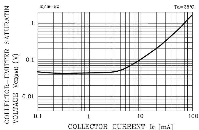
Fig. 2 V_{CE(SAT)} - I_C
